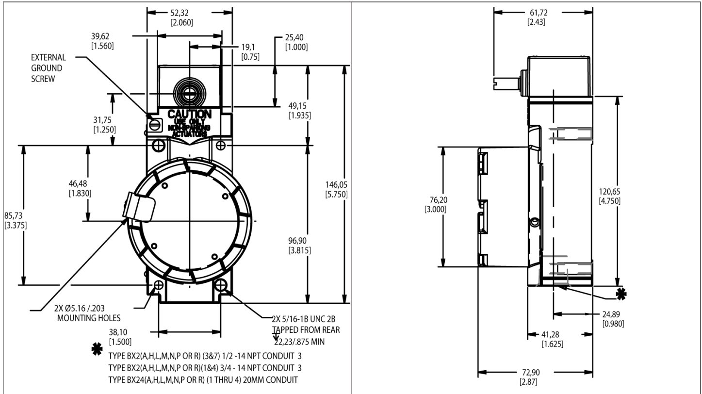
FIGURE 8. SIDE ROTARY MOUNTING DIMENSIONS (For reference only) mm/in FIGURA 8. DIMENSIONES DE MONTAJE DE ROTACIÓN LATERAL (solo como referencia) mm/pulgadas FIGURE 8. ROTATIF LATERAL - COTES DE MONTAGE (à titre indicatif uniquement) mm/in FIGURA 8. DIMENSIONI DI MONTAGGIO DELLA ROTELLA LATERALE (solo di riferimento) mm/in ABBILDUNG 8: SEITLICHER SCHWENKHEBEL EINBAUMASSE – nur als Richtwerte (mm/Zoll) FIGURA 8. DIMENSÕES DA MONTAGEM GIRATÓRIA LATERAL (apenas para referência) mm/in 图8. 侧面旋转式安装尺寸 (仅供参考) mm/in РИСУНОК 8. КРЕПЕЖНЫЕ РАЗМЕРЫ ДЛЯ БОКОВОГО ПОВОРОТНОГО РЫЧАГА (только для справки), мм/дюймы
