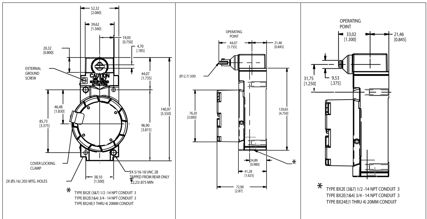
FIGURE 9. FRONT ROLLER PLUNGER MOUNTING DIMENSIONS (For reference only) mm/in FIGURA 9. DIMENSIONES DE MONTAJE DE ÉMBOLO DE RODILLO FRONTAL (solo como referencia) mm/pulgada FIGURE 9. POUSSOIR A GALET AVANT - COTES DE MONTAGE (à titre indicatif uniquement) mm/in FIGURA 9. DIMENSIONI DI MONTAGGIO DEL PULSANTE A ROTELLA ANTERIORE (solo di riferimento) mm/in ABBILDUNG 9: ABBILDUNG 8: VORDERER ROLLENSTÖSSEL EINBAUMASSE – nur als Richtwerte (mm/Zoll) FIGURA 9. DIMENSÕES DE MONTAGEM DO ÊMBOLO FRONTAL COM ROLDANA (apenas para referência) mm/in 图9. 前部滚轮柱塞安装尺寸 (仅供参考) mm/in РИСУНОК 9. КРЕПЕЖНЫЕ РАЗМЕРЫ ДЛЯ ПЕРЕДНЕГО РОЛИКОВОГО ПЛУНЖЕРА (только для справки), мм/дюймы
