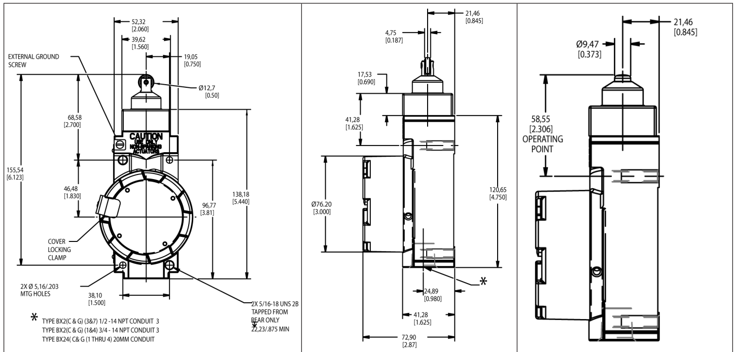
FIGURE 10. TOP ROLLER PLUNGER MOUNTING DIMENSIONS (For reference only) mm/in FIGURA 10. DIMENSIONES DE MONTAJE DE ÉMBOLO DE RODILLO SUPERIOR (solo como referencia) mm/pulgada FIGURE 10. POUSSOIR A GALET SUPERIEUR - COTES DE MONTAGE (à titre indicatif uniquement) mm/in FIGURA 10. DIMENSIONI DI MONTAGGIO DEL PULSANTE A ROTELLA SUPERIORE (solo di riferimento) mm/in ABBILDUNG 10: OBERER ROLLENSTÖSSEL EINBAUMASSE – nur als Richtwerte (mm/Zoll) FIGURA 10. DIMENSÕES DE MONTAGEM DO ÊMBOLO SUPERIOR COM ROLDANA (apenas para referência) mm/in 图10. 顶部滚轮柱塞安装尺寸 (仅供参考) mm/in РИСУНОК 10. КРЕПЕЖНЫЕ РАЗМЕРЫ ДЛЯ ВЕРХНЕГО РОЛИКОВОГО ПЛУНЖЕРА (только для справки), мм/дюймы
